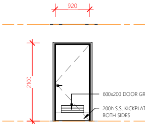
DOOR TYPE F
