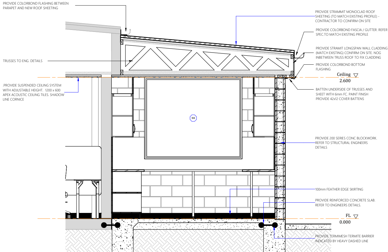
Section A1
