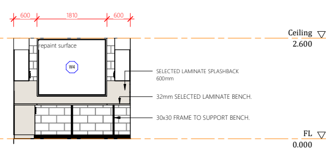
Elevation 1B 1 : 50
