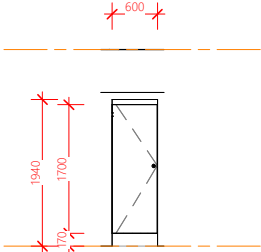
DOOR TYPE H
