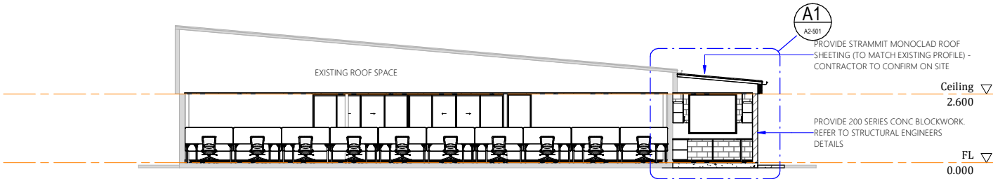
Section A 1 : 100
