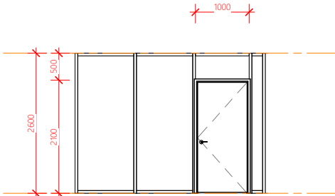
DOOR TYPE B
