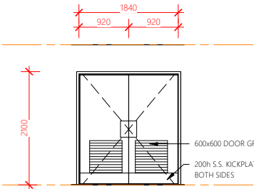
DOOR TYPE J
