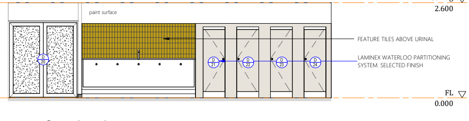
Elevation 5B
