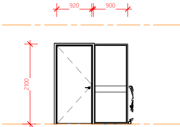
DOOR TYPE E
