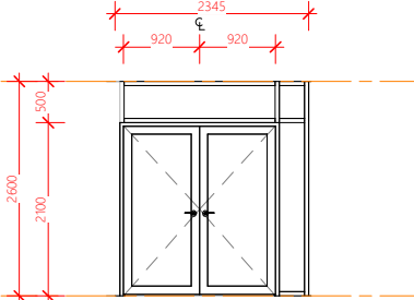
DOOR TYPE C
