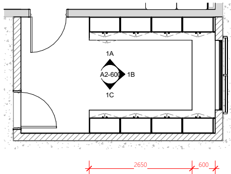
Internal Plan 1 1 : 50
