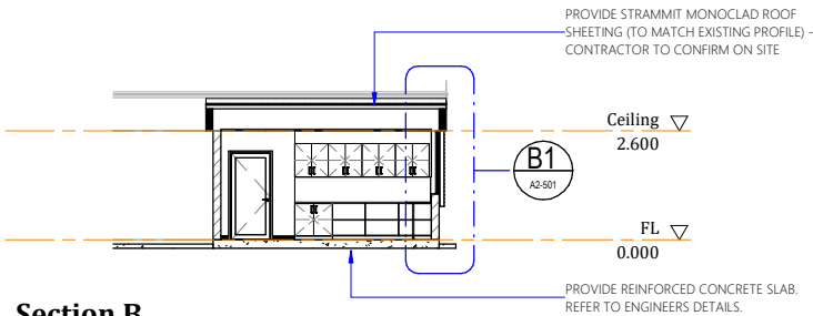
Section B 1 : 100
