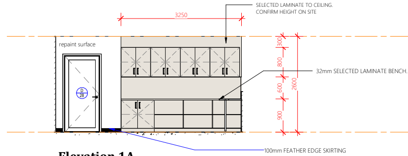
Elevation 1A 1 : 50
