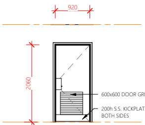
DOOR TYPE G
